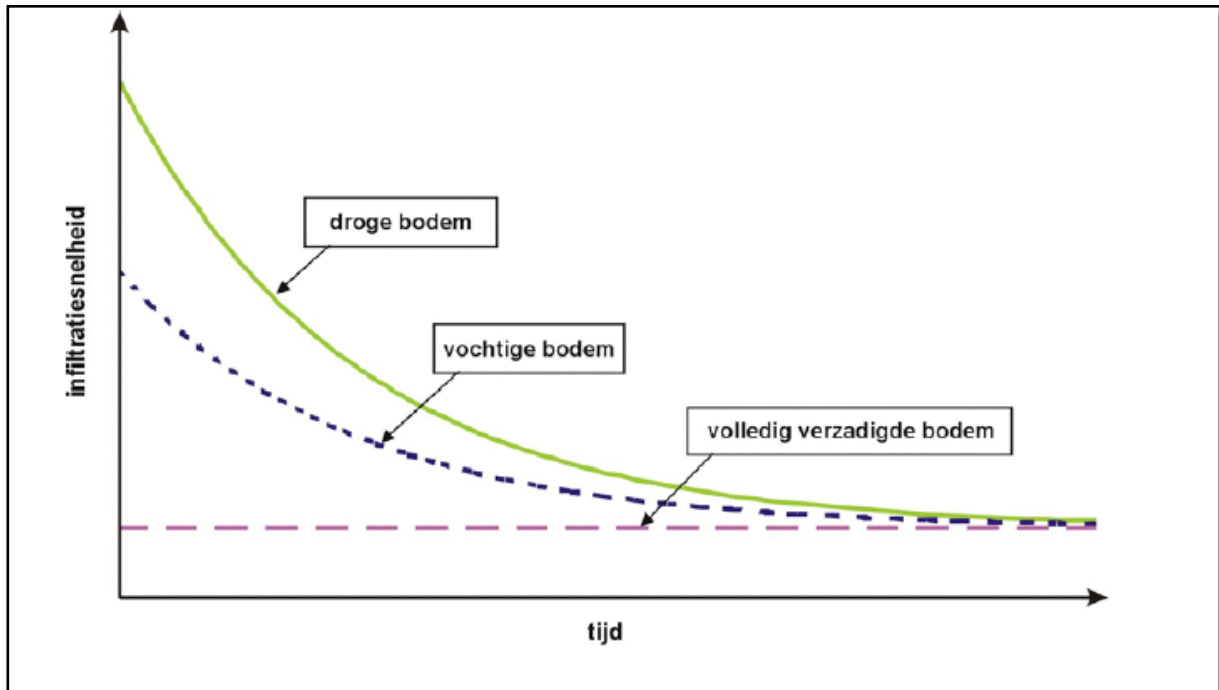
Figuur 2: Infiltratiesnelheid met verschillende initiële watergehaltes
