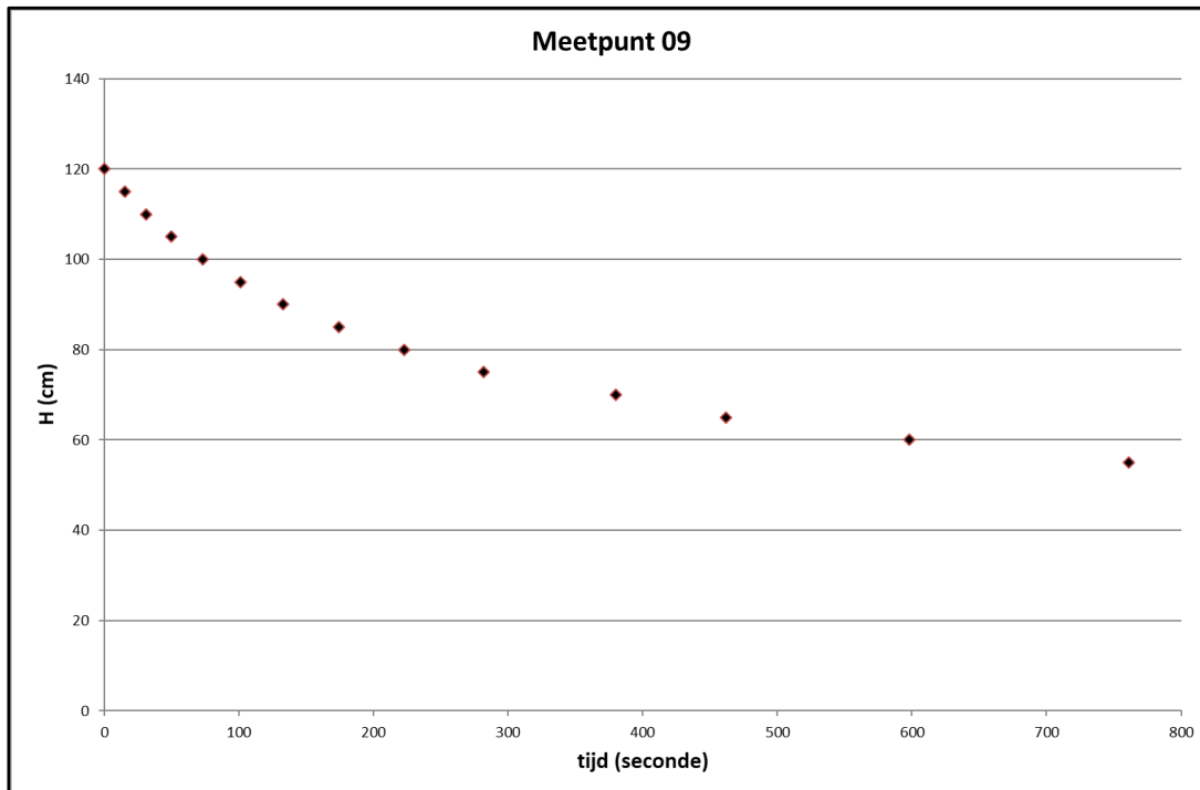
Figuur 3: relatie kolomhoogte en verstreken tijd
