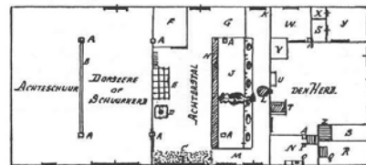
PLATTEGROND. A. STANDERS, B. MILKRIJK, C. STALMEST, D. HOUWING, E. HEINENHOORT, F. VARKENKOP, G. PARRDESTAL, H. ZOEI, J. KOESTAL, K. NODINGAL, L. SOKPTEL, M. GENGSKER, N. DE GEUT, O. GEUISTEN, P. TRAP VAN GEUT NAAR OPMER, Q. TRAP NAAR OPMER TOEGANG NAAR VELD, R. TRAP NAAR TOLDER, R. OPMER, W. RANER, X. KLEERKAST, Y. T. KEMMERKE. v.d.
