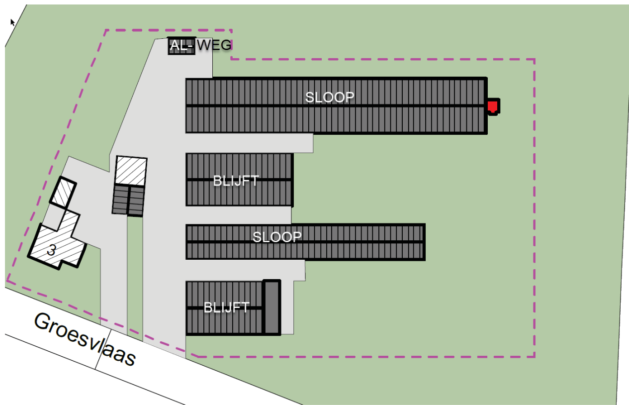
Figuur 2. Tekening met gewenste aanpassingen (Bron: Agra-Matic)
