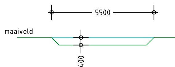
Doorsnede wadi
