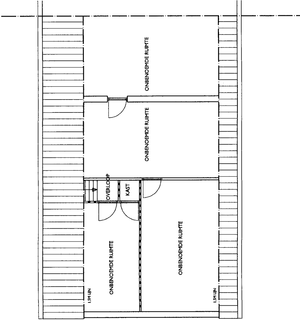
VERDIEPING - NIEUW -
