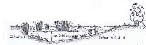
Doorsnede wadi
