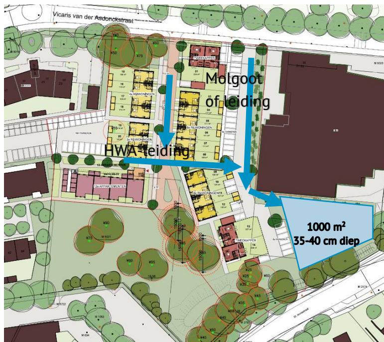
Afbeelding 5: voorstel hemelwaterverwerking binnen Fitland
